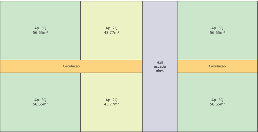
Pavimento Tipo 2 2Q + 4 3Q (11x)
